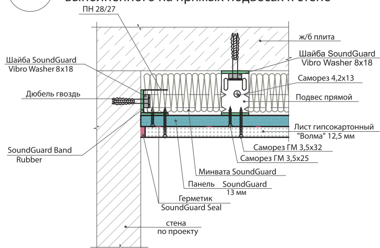
4.1.1.a Узел примыкания звукоизолирующего потолка, выполненного на прямых подвесах к стене
