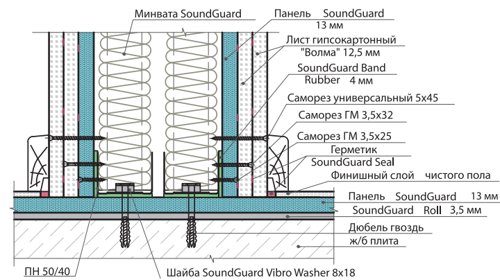
1.2.2.г Узел примыкания звукоизолирующей перегородки на двойном металлическом каркасе к полу с панелью SoundGuard
