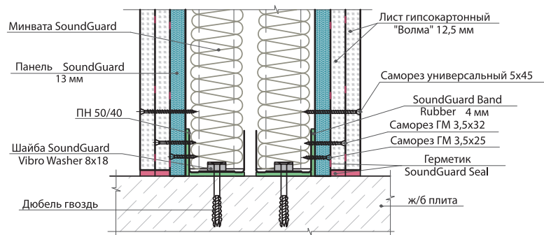
1.2.2.м Узел сопряжения звукоизолирующих перегородок на двойном металлическом каркасе
