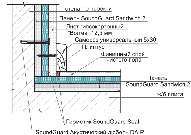
2.2.1.п Узел примыкания стены с бескаркасной обшивкой панелью SoundGuard Sandwich 2 к стене с каркасной обшивкой на виброизоляционном креплении
