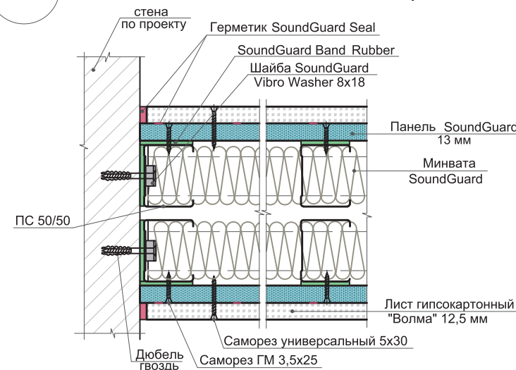
Узел примыкания звукоизолирующей перегородки на двойном металлическом каркасе к стене
