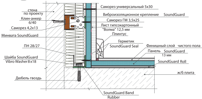
5.1.1.д Узел примыкания звукоизолирующего пола и каркасной обшивки стены
