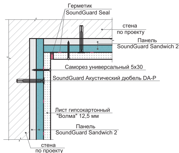
2.2.1.з Узел сопряжения стен с бескаркасной обшивкой панелью SoundGuard Sandwich 2
