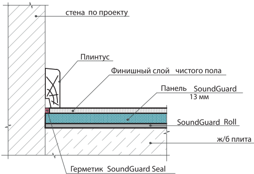
5.1.1.a Узел примыкания звукоизолирующего пола к стене
