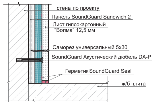
2.2.1.a 2.2.1.б Узел примыкания бескаркасной обшивки стены панелью SoundGuard Sandwich 2 к межэтажному перекрытию
