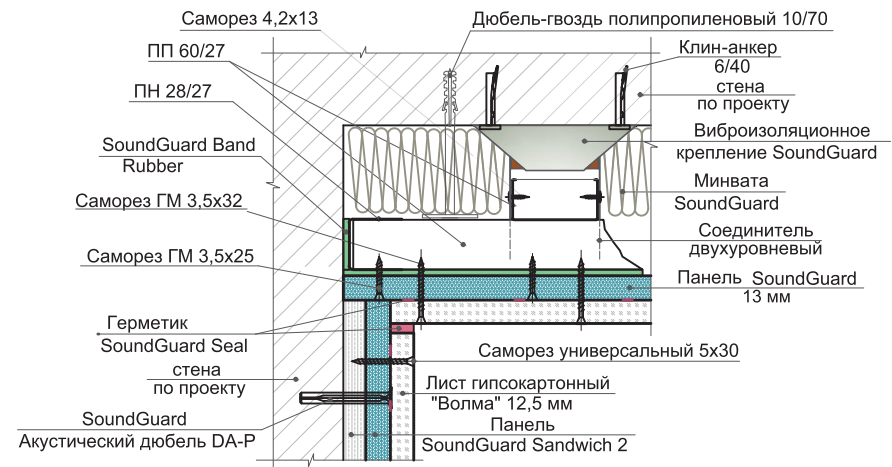
2.2.1.п Узел примыкания стены с бескаркасной обшивкой панелью SoundGuard Sandwich 2 к стене с каркасной обшивкой на виброизоляционном креплении
