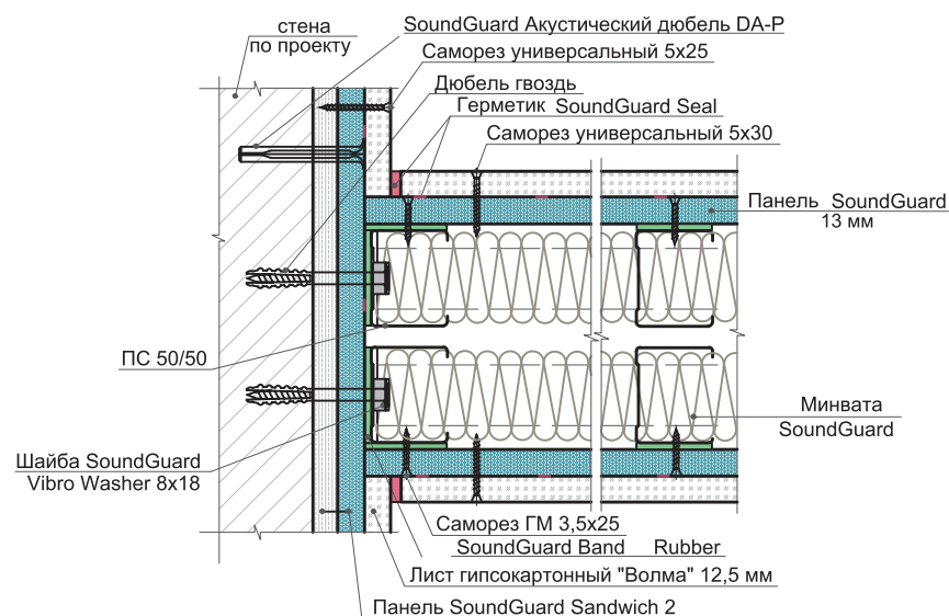
Узел примыкания звукоизолирующей перегородки на двойном металлическом каркасе к стене с обшивкой SoundGuard Sandwich 2
