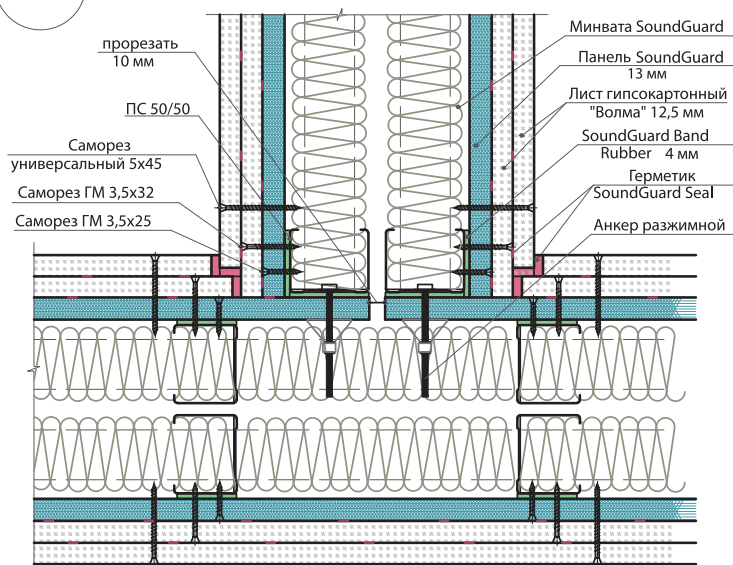
1.2.2.м Узел сопряжения звукоизолирующих перегородок на двойном металлическом каркасе
