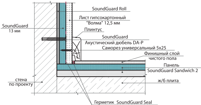
5.2.1.б Узел примыкания звукоизолирующего пола и бескаркасной обшивки стены
