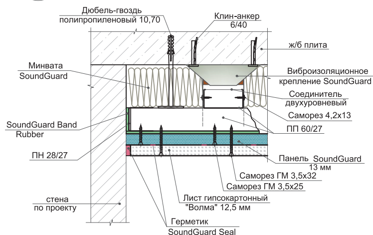
4.2.1.a Узел примыкания звукоизолирующего потолка, выполненного на звукоизоляционных креплениях SoundGuard, к стене
