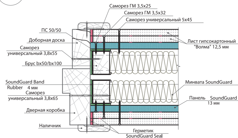
1.2.2.с Узел примыкания звукоизолирующей перегородки на двойном металлическом каркасе к дверной коробке
