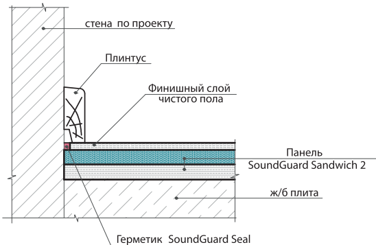
5.2.1.a Узел примыкания звукоизолирующего пола к стене
