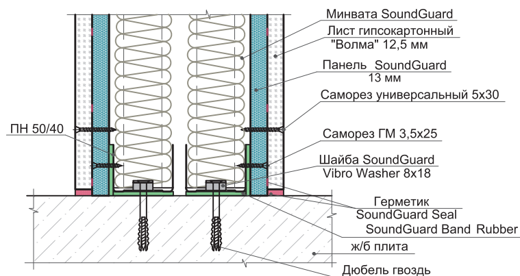
Узел примыкания звукоизолирующей перегородки на двойном металлическом каркасе к стене с обшивкой SoundGuard Sandwich 2
