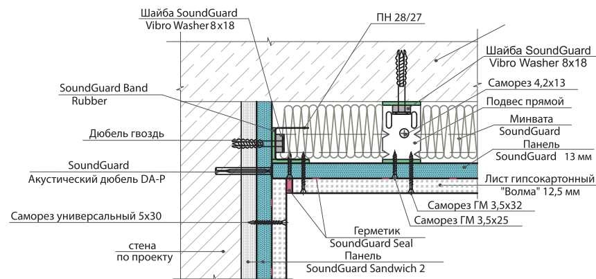
4.1.1.в Узел примыкания звукоизолирующего потолка, выполненного на прямых подвесах, к стене с обшивкой SoundGuard Sandwich 2
