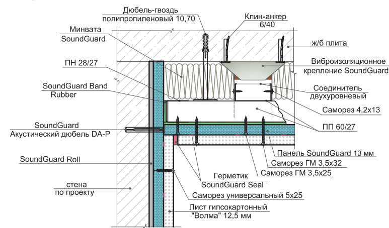
4.2.1.б Узел примыкания звукоизолирующего потолка, выполненного на звукоизоляционных креплениях SoundGuard, к стене с обшивкой панелью SoundGuard
